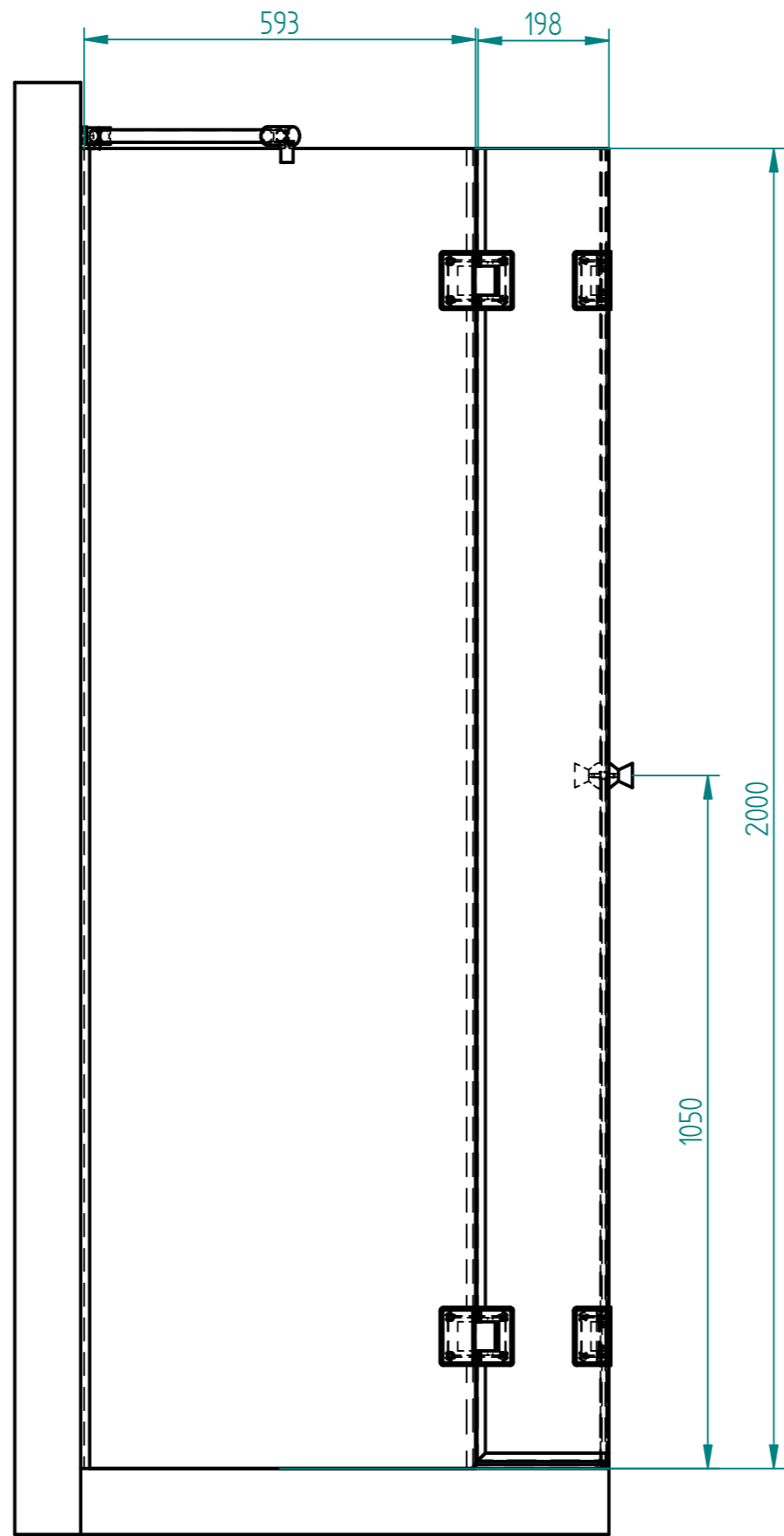
EINZELHEIT A 1:2
